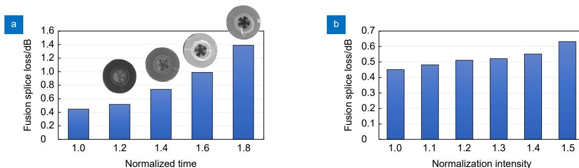
图 3 不同熔接参数对损耗的影响。(a) 放电时间对熔接损耗的影响；(b) 放电强度对熔接损耗的影响
