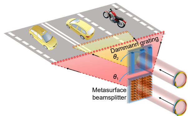
图 1 设计的超构表面分束器和达曼光栅的概念示意图
