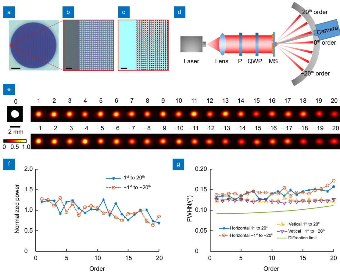
图 4 (a, b) 加工的超构表面的光学显微镜图像。(a) 5 倍物镜, 比例尺为 200\ \mu\text{m} ; (b) 100 倍物镜, 比例尺为 2\ \mu\text{m} ; (c) (b) 超构表面相同区域的设计图纸, 比例尺为 2\ \mu\text{m} ; (d) 实验光路示意图, P、QWP、MS 分别表示偏振片, 四分之一波片和超构表面; (e) 相机采集的不同衍射级次的 41 束光斑。每个光斑裁切为 3\ \text{mm} 大小的方块后拼接在一起; (f) 实验测得的光斑功率。蓝色星标为 1 至 20 级光斑, 橙色圆标为 -1 至 -20 级光斑; (g) 实验测得的光斑半高全宽。蓝色星标实线和橙色圆标点线分别为 1 至 20 级和 -1 至 -20 级的水平方向半高全宽。黄色正三角形虚线和紫色倒三角形点线分别为 1 至 20 级和 -1 至 -20 级的竖直方向半高全宽。绿色实线为光斑横向的衍射极限
