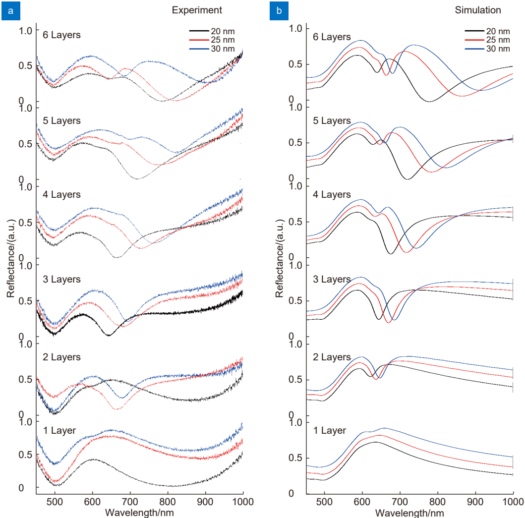
图 4 不同直径的 (20 nm (黑色曲线)、25 nm (红色曲线)、30 nm (蓝色曲线)) 金纳米颗粒超晶格薄膜不同层数的反射光谱。 (a) 实验测量结果; (b) 数值计算结果
