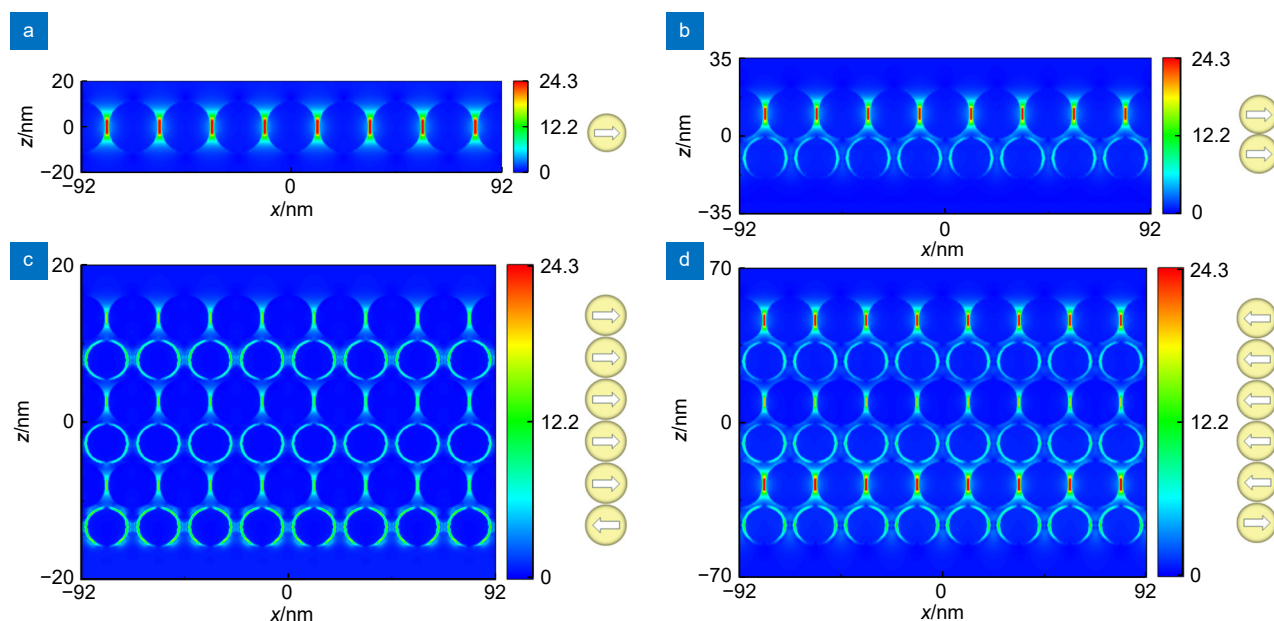
图3 直径为20 nm, 颗粒间间隔为1 nm的金纳米颗粒薄膜近场分布图: (a) 单层; (b) 双层; (c) 六层 ( \lambda=638 nm); (d) 六层 ( \lambda=778 nm)。在旁边展示了通过纳米颗粒内部的电流分布分配等离子体模式, 每层颗粒中的偶极矩由白色箭头指示
