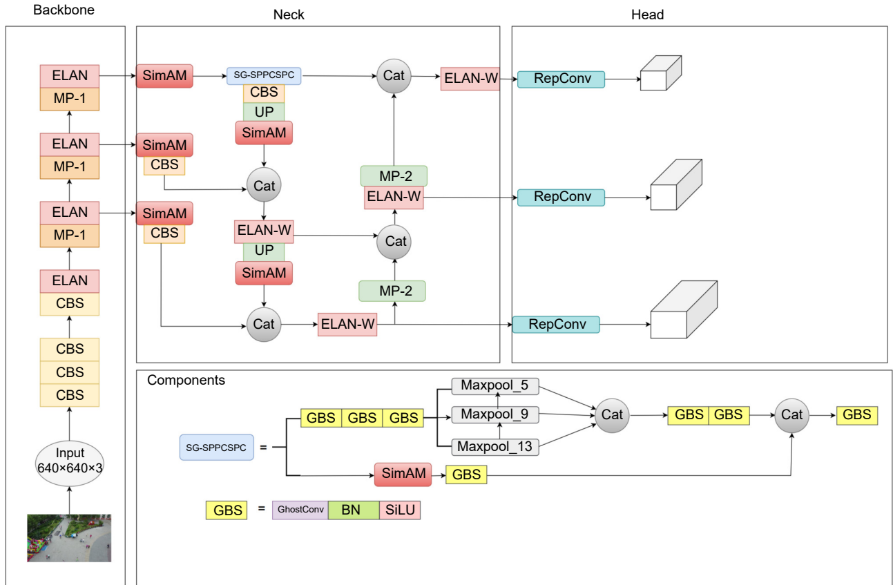
图2 SSG-YOLOv7 整体结构
