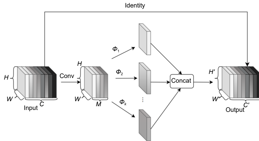
图3 GhostConv 结构图
