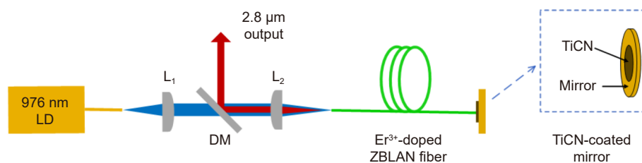
图 2 TiCN 作为 SA 的被动 QSML 掺铒氟化物光纤激光器实验装置图
