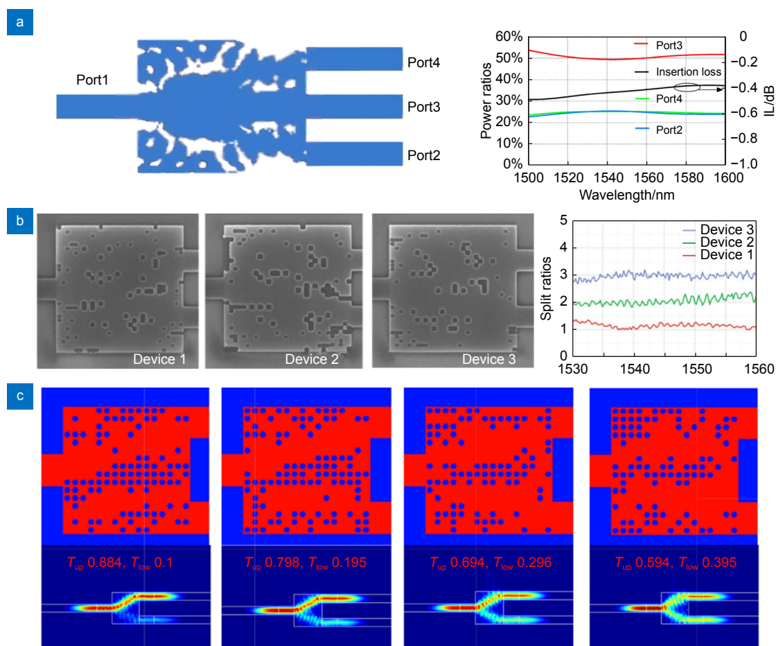
图 5 任意分束比功率分束器的结构和性能。(a) 分束比为 1:2:1 的 1 \times 3 功率分束器 [67] ; (b) 分束比分别为 1:1、1:2 和 1:3 的 1 \times 2 功率分束器 [63] ; (c) 分束比分别为 9:1、8:2、7:3 和 6:4 的 1 \times 2 功率分束器 [88]
