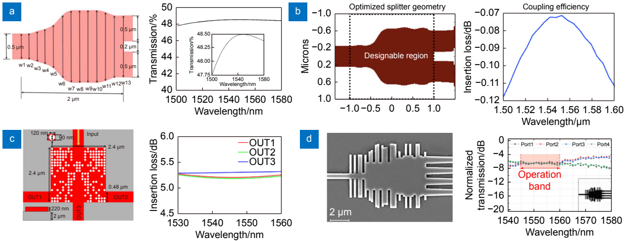
图 3 单个器件的多通道功率分束器的结构与性能。(a) 和 (b) 1 \times 2 功率分束器 [75,79] ; (c) 1 \times 3 功率分束器 [86] ; (d) 1 \times 4 功率分束器 [62]
