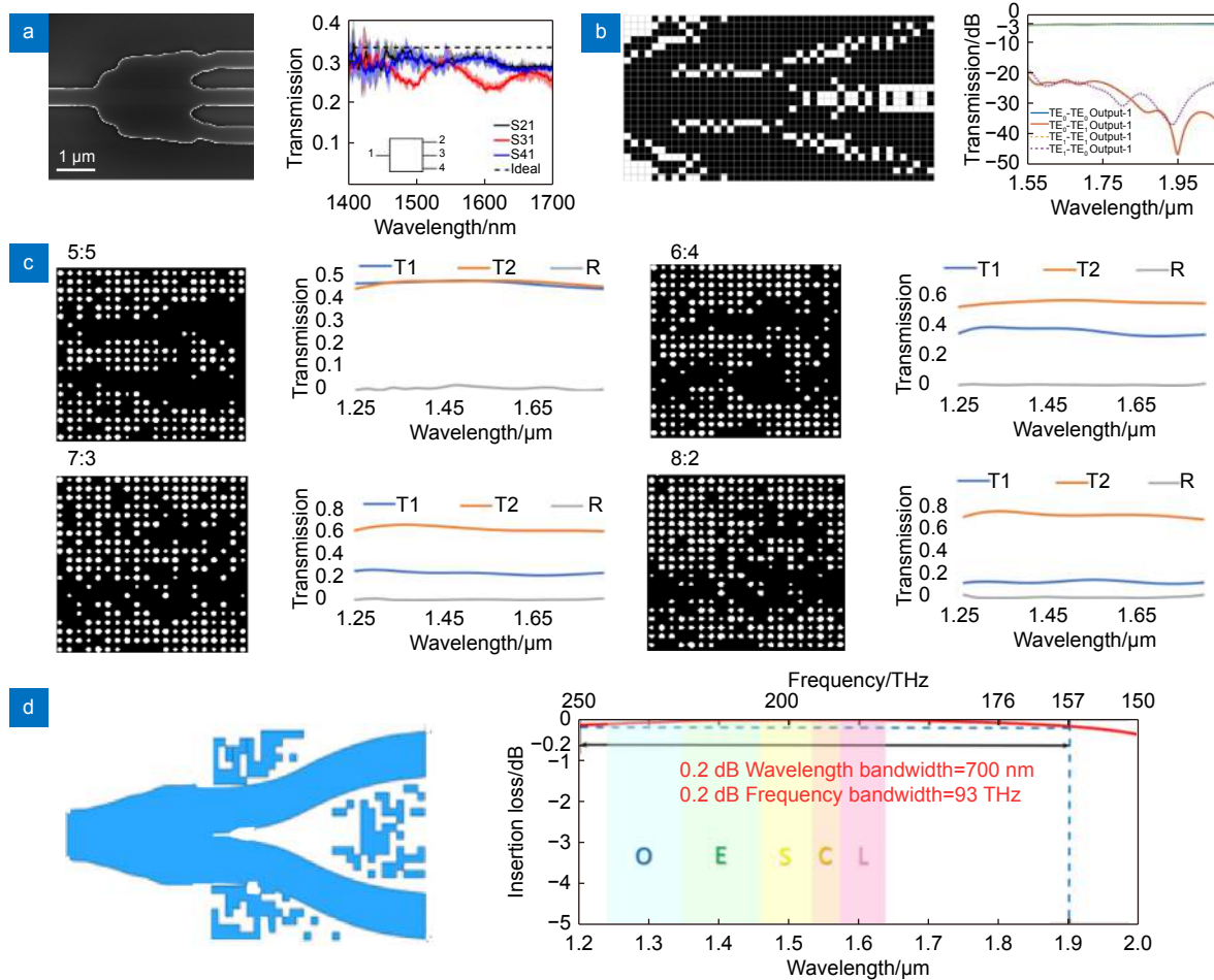
图 10 宽带功率分束器的结构和性能。(a) 300 nm 带宽的 1×4 功率分束器 [96] ；(b) 445 nm 带宽的 1×2 功率分束器 [97] ；(c) 550 nm 带宽的 1×2 功率分束器 [98] ；(d) 700 nm 带宽的 1×2 功率分束器 [71]
