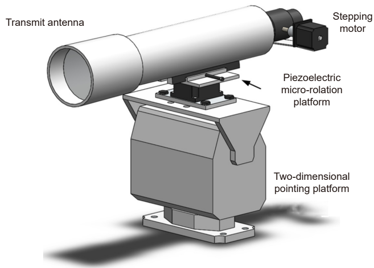
图 4 粗精分级控制系统 [42-43]
