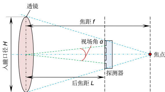
图 5 阵列探测器视场原理图
