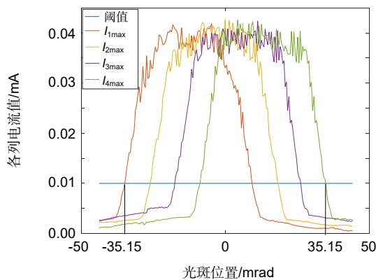
图 12 粗跟踪视场实验图
