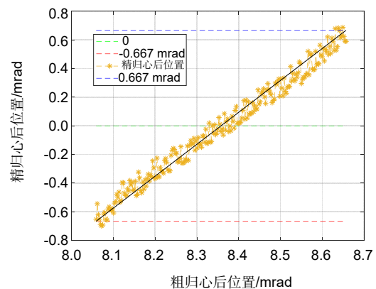
图 10 精归心后光斑位置折线图
