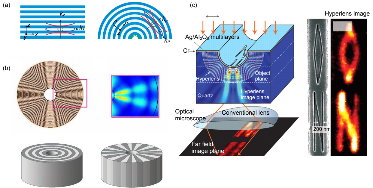
图 4 (a) 基于金属介质多层膜的平板形和圆柱形双曲超材料及其各自色散曲线 [47] . (b) 上图: 双曲超透镜结构示意图及仿真结果. 下图: 双曲超透镜的两种设计思路, 切向层叠和径向层叠 [6] . (c) 左图: 超透镜结构示意图, 入射波长 365 nm; 右图: 字母“ON”的超越衍射极限图样 [7] .
