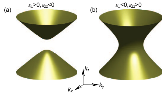
图1 双曲超材料中横磁波的等频率面 [13] 。
