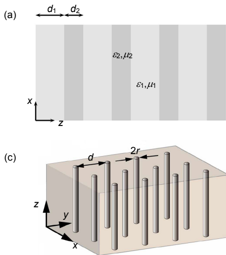
图 2 (a) 金属-介质多层膜结构示意图, \epsilon 、 \mu 、 d 分别代表材料的介电常数、磁导率和薄膜厚度 [20] 。(b) 半导体多层膜结构有效介电常数的实部图, \epsilon_{\perp} 、 \epsilon_{\parallel} 分别表示垂直和平行于多层膜的介电常数 [15] 。(c) 金属纳米线阵列结构示意图, d 为金属纳米线阵列周期, r 为金属纳米线半径 [16] 。
