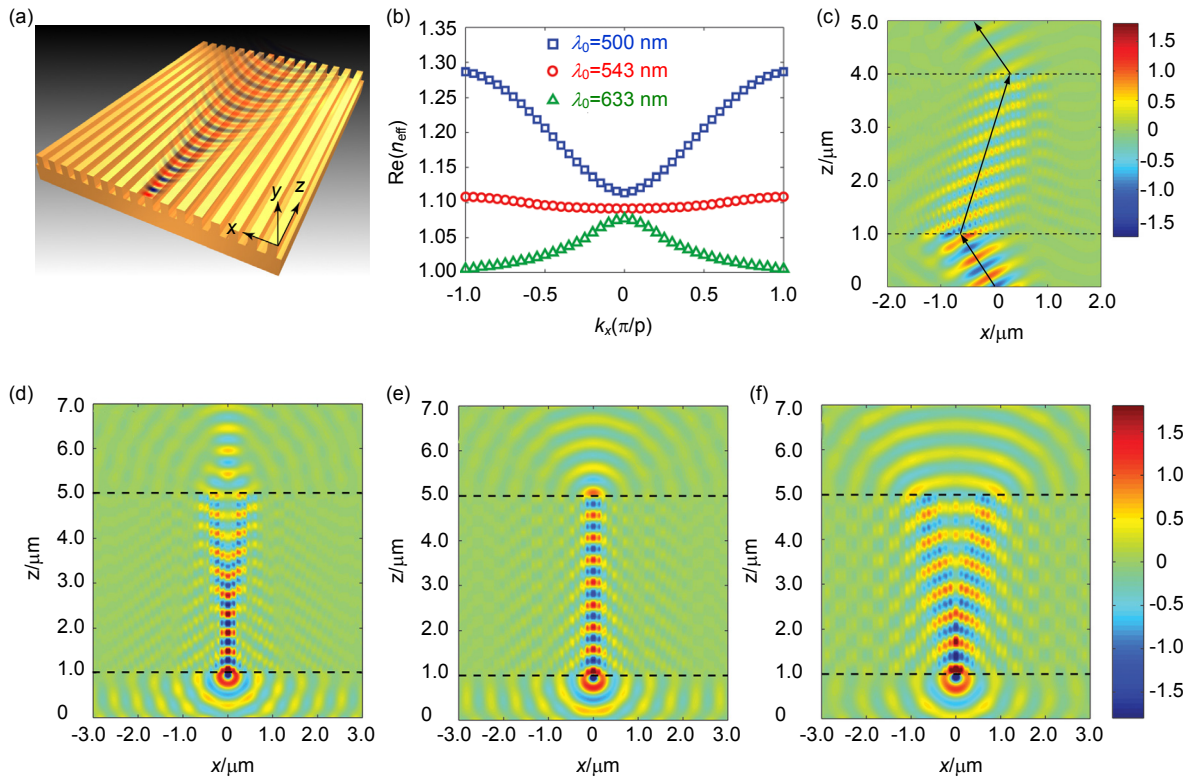
图 7 (a) 基于光栅结构的超表面结构示意图 [74] . (b) 光栅在不同入射光下的色散分布图, 光栅周期 120 nm, 宽度 60 nm, 高度 80 nm [74] . (c) 光栅超表面的负折射效应, 入射波长 500 nm, 光栅周期 100 nm, 宽度 40 nm, 高度 100 nm [74] . (d)~(f) 入射波长分别为 500 nm(左), 543 nm(中), 633 nm(右)时结构表面等离子元波传播 [74] .
