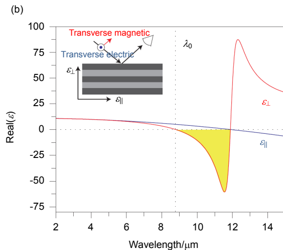
图 2 (a) 金属-介质多层膜结构示意图, \epsilon 、 \mu 、 d 分别代表材料的介电常数、磁导率和薄膜厚度 [20] 。(b) 半导体多层膜结构有效介电常数的实部图, \epsilon_{\perp} 、 \epsilon_{\parallel} 分别表示垂直和平行于多层膜的介电常数 [15] 。(c) 金属纳米线阵列结构示意图, d 为金属纳米线阵列周期, r 为金属纳米线半径 [16] 。
